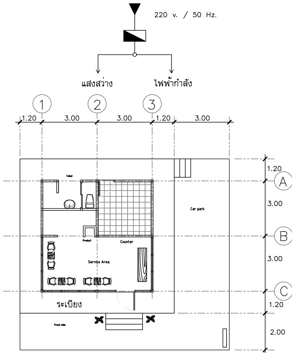
หมายเหตุ 1 แบบวงจรสายเดี่ยว (One Line Diagram)
